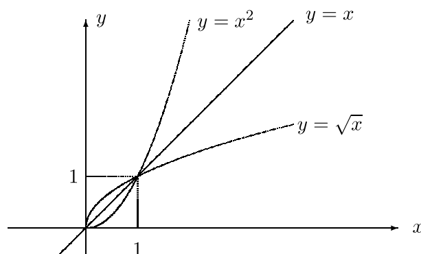
Figura 2.8: Gráficos de y = x , y = x^2 y y = \sqrt{x}
