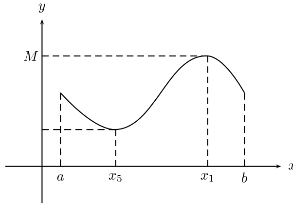
Figura 2.34: Teorema de Weierstrass
