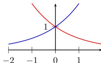
(a) En azul 2^x . En rojo 2^{-x}
