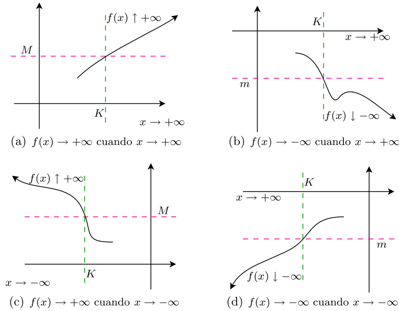
Figura 2.13: Casos posibles de límites infinitos si |x| \rightarrow +\infty
