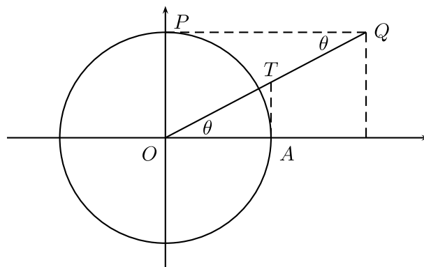
Figura 3.14: La función y = \operatorname{cosec} x
