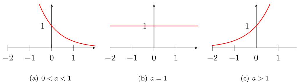
Figura 3.40: Gráfico de a^x .
