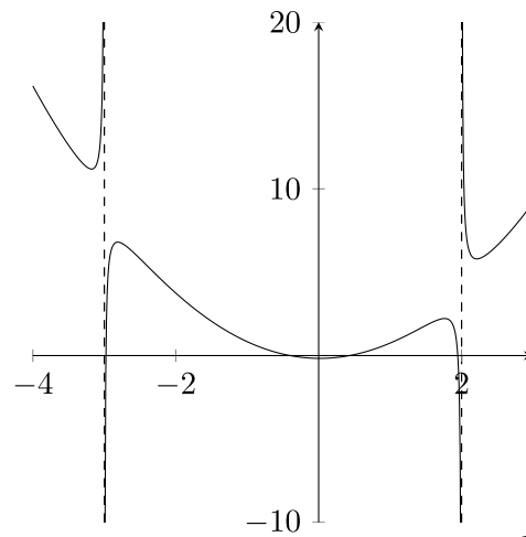
Figura 2.26: Gráfico de g(x) = x^2 + \frac{1}{x^2 + x - 6}
