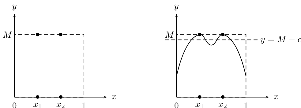
Figura 2.40: La función f no puede ser continua
