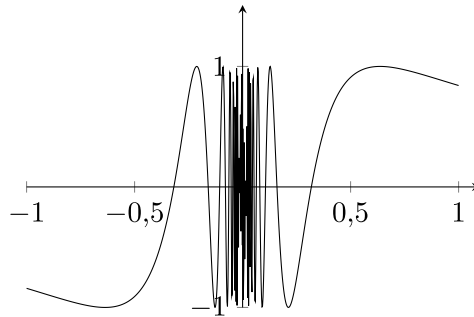
Figura 3.34: Gráfico de f(x) = \sin \frac{1}{x}
