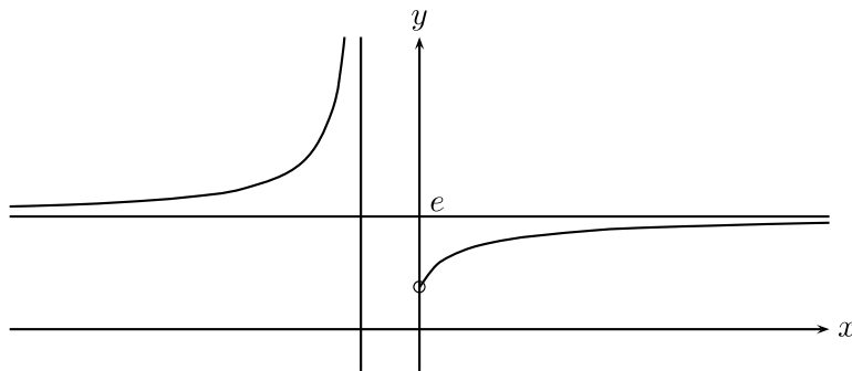
Figura 3.41: Gráfico de \left(1 + \frac{1}{x}\right)^x
