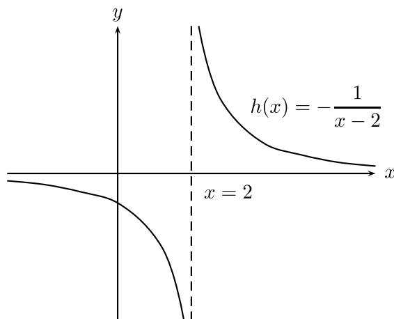
Figura 2.18: Gráfico de h(x) = -\frac{1}{x-2}
