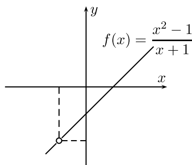
Figura 2.22: Existencia del límite sin que la función esté definida en el punto
