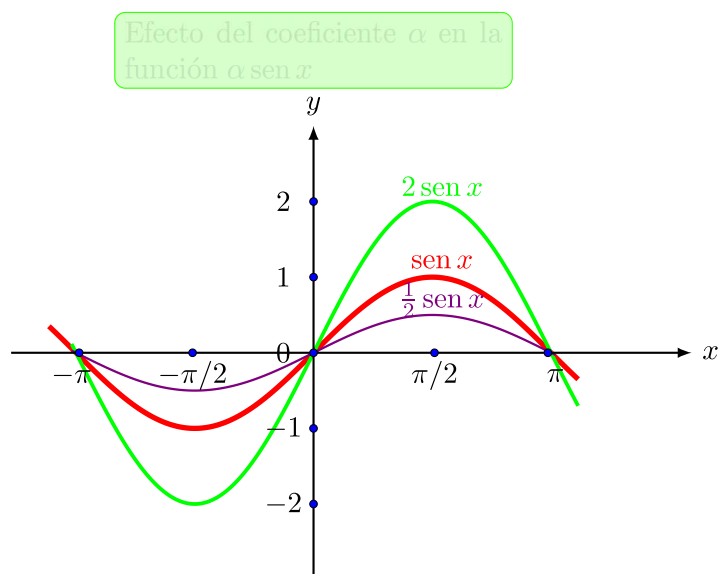
Figura 3.20: Efecto del coeficiente \alpha en la función \alpha \operatorname{sen} x
