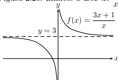
Figura 2.21: Asíntota horizontal de f(x) = \frac{3x + 1}{x}
