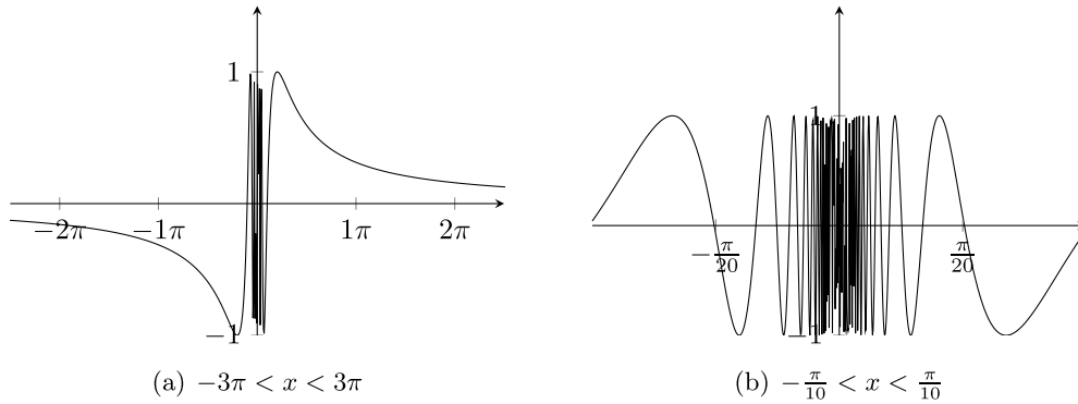
Figura 3.32: Gráfico de f(x) = \sin \frac{1}{x}
