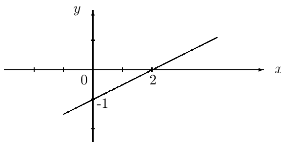
Figura 2.3: Gráfico de f(x) = \frac{1}{2}x - 1
