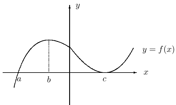
Figura 2.12: Gráfico de f invertible
