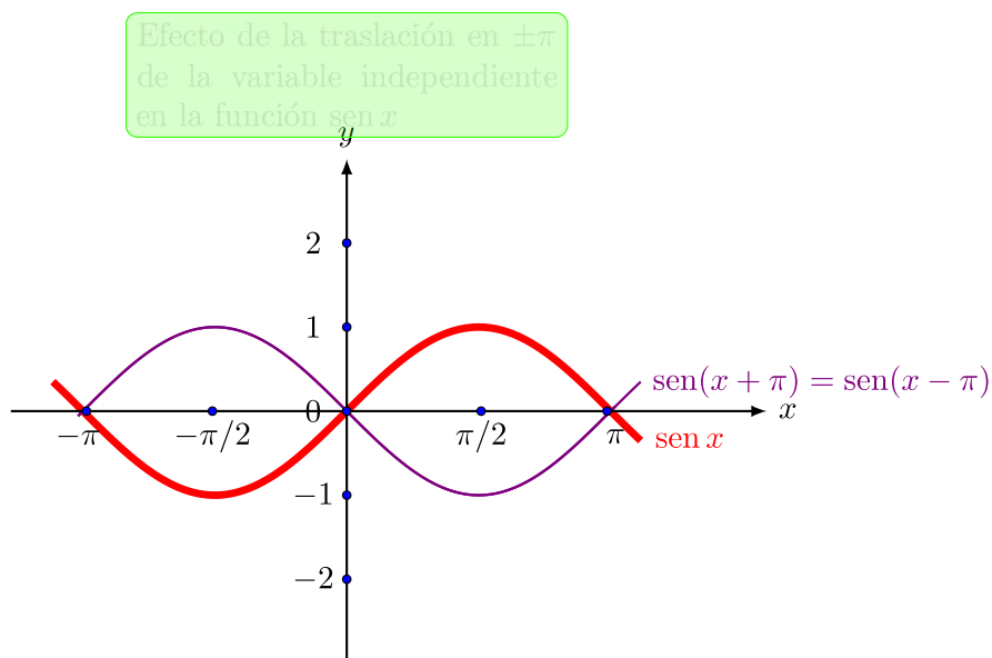
Figura 3.21: Efecto de la traslación en \pm\pi de la variable independiente en la función \operatorname{sen} x
