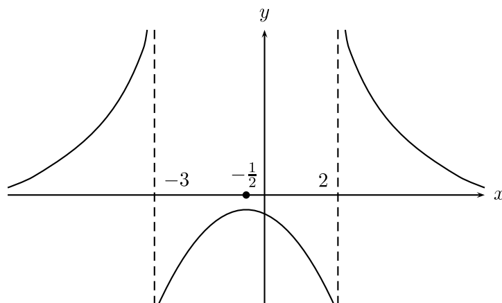
Figura 2.25: Gráfico de f(x) = \frac{1}{x^2 + x - 6}
