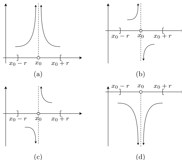
Figura 2.15: Límites infinitos en una vecindad de x_0 .
