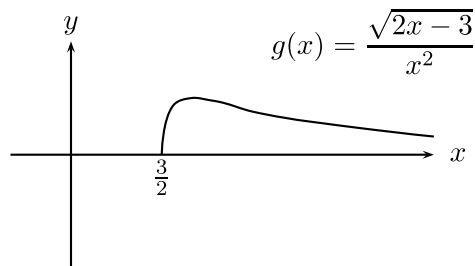
Figura 2.28: Gráfico de g(x) = \frac{\sqrt{2x-3}}{x^2}
