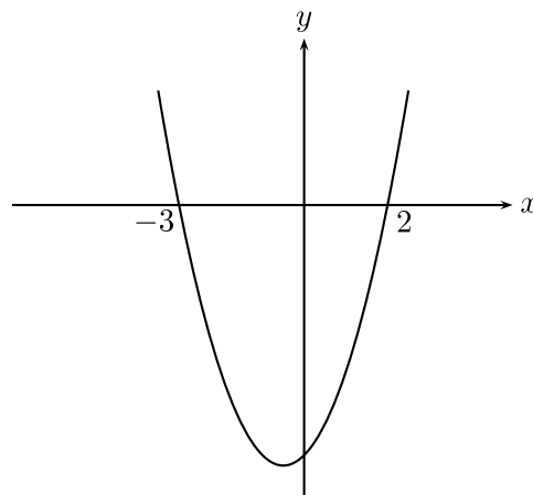
Figura 2.24: Gráfico de y = x^2 + x - 6
