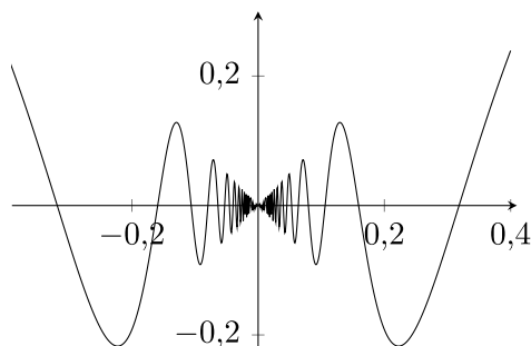
Figura 3.35: Gráfico de f(x) = x \sin \frac{1}{x}
