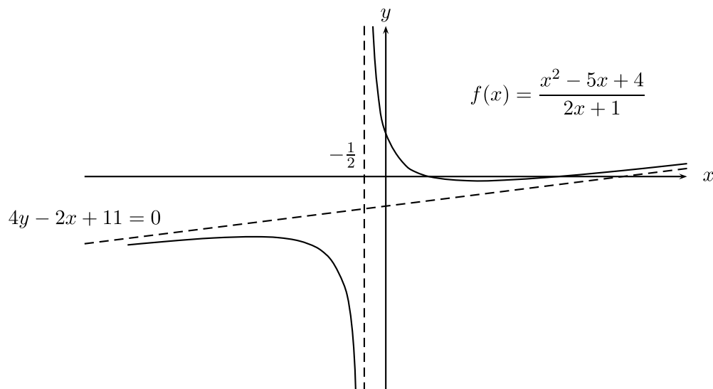
Figura 2.30: Gráfico de f(x) = \frac{x^2 - 5x + 4}{2x + 1}
