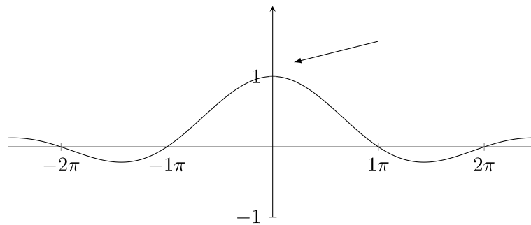
Figura 3.31: y = \frac{\operatorname{sen} x}{x} . Observar que \lim_{x \rightarrow 0} f(x) = 1
