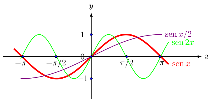
Figura 3.19: Efecto del coeficiente \omega en la función \text{sen}(\omega x)
