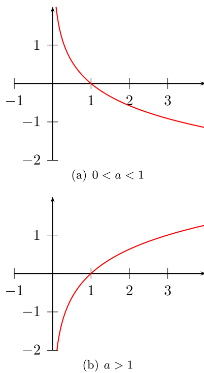
Figura 3.43: Gráfico de \log_a(x) .
