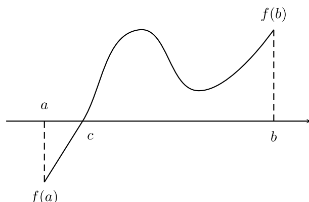
Figura 2.33: Teorema de Bolzano - Weierstrass
