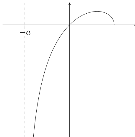
Figura 2.11: Una rama de la estrofoide
