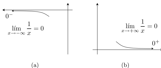
Figura 2.20: Límites a \pm\infty de \frac{1}{x} .
