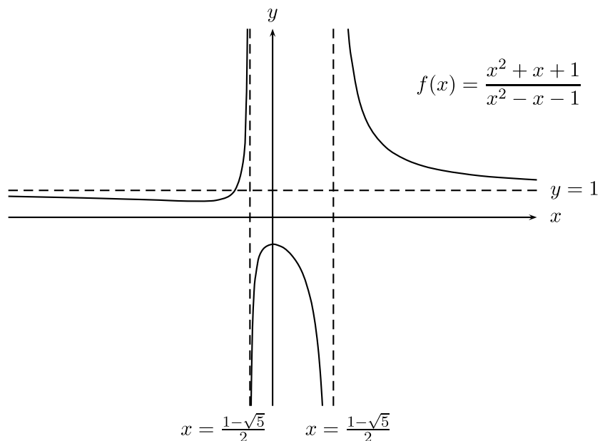
Figura 2.29: Gráfico de f(x) = \frac{x^2 + x + 1}{x^2 - x - 1}
