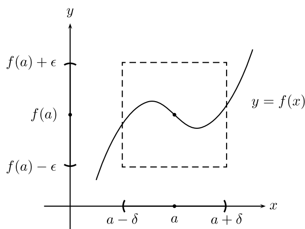
Figura 2.31: Interpretación geométrica de la continuidad
