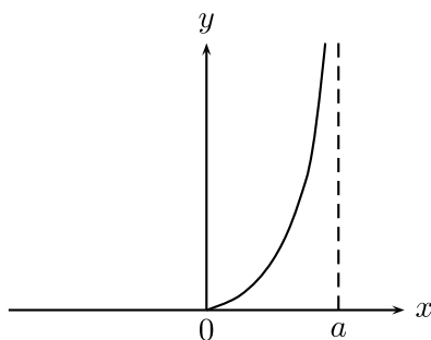
Figura 2.10: Una rama de la cisoide
