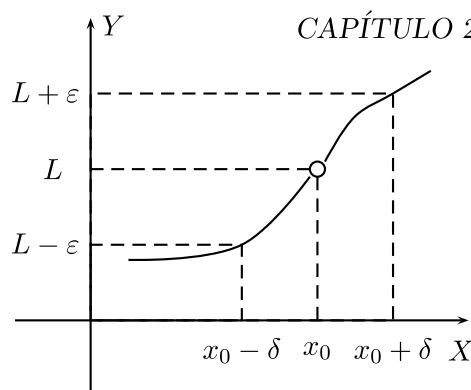
Figura 2.23: Interpretación geométrica del límite
