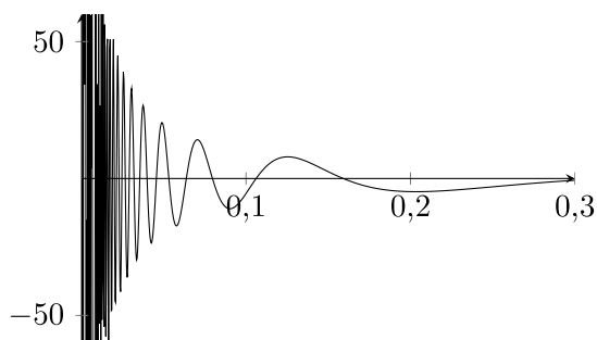
Figura 3.36: Gráfico de h(x) = \frac{1}{x} \sin \frac{1}{x}
