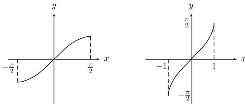
Figura 3.37: La función \sin x y su inversa
