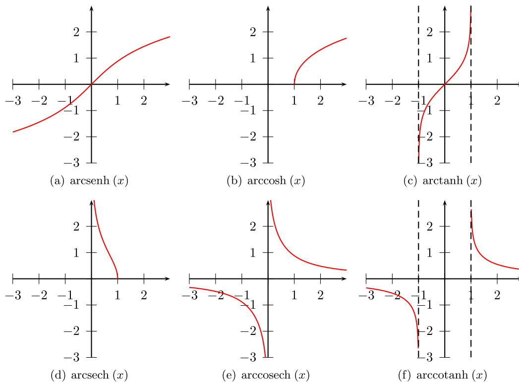
Figura 3.45: Funciones hiperbólicas inversas
