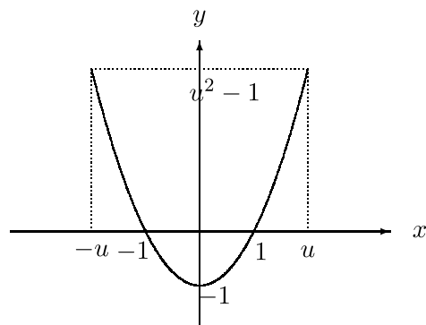
Figura 2.4: Gráfico de f(x) = x^2 - 1
