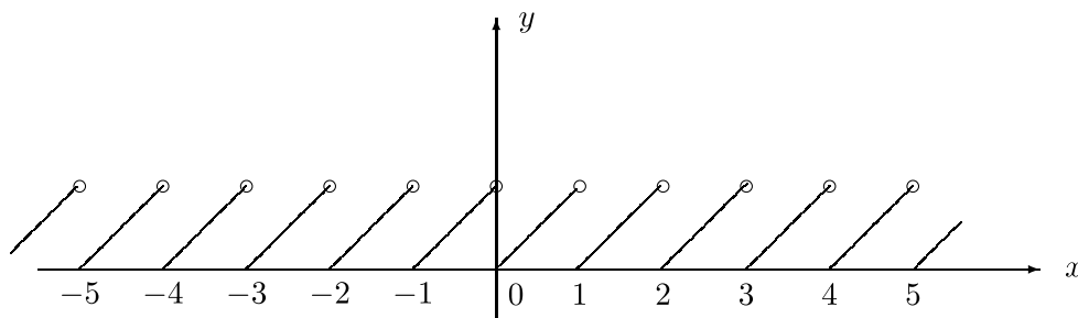
Figura 2.5: Gráfico de f(x) = x - [x]
