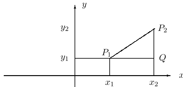
Figura 3.1: Distancia entre dos puntos
