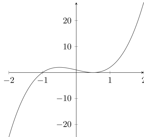
Figura 2.19: Gráfico de f(x) = 4x^3 - 3x + 1
