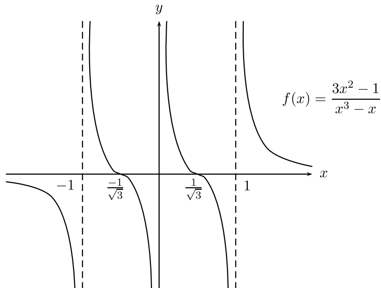
Figura 2.27: Gráfico de f(x) = \frac{3x^2 - 1}{x^3 - x}
