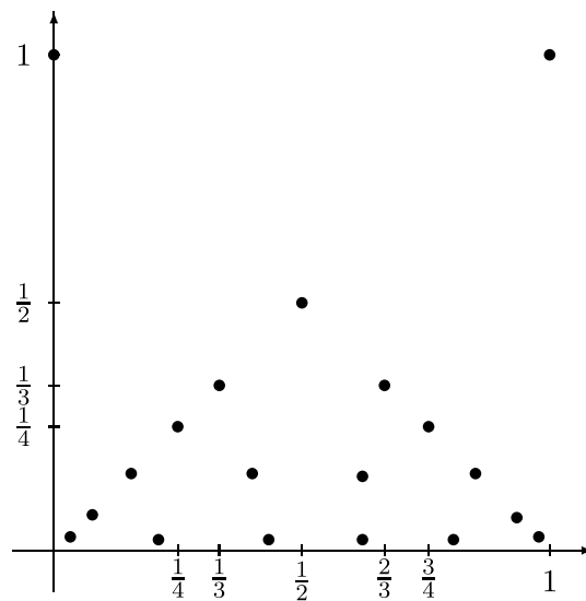
Figura 2.7: Gráfico de g
