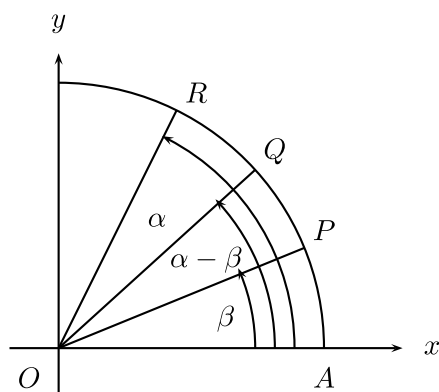
Figura 3.16: Diagrama de Cauchy Donde:
