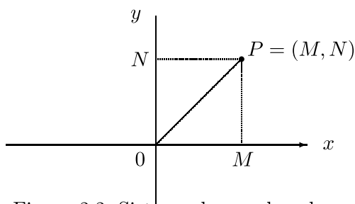
Figura 2.2: Sistema de coordenadas rectangulares
