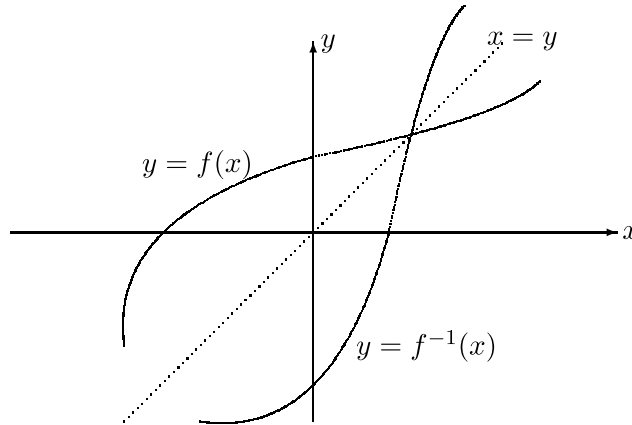
Figura 2.6: Gráfico de f y su inversa f^{-1}
