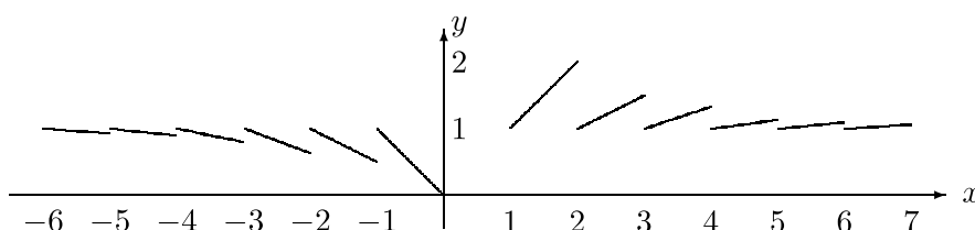
Figura 2.9: Gráfico de la función f(x) = \frac{x}{[x]}
