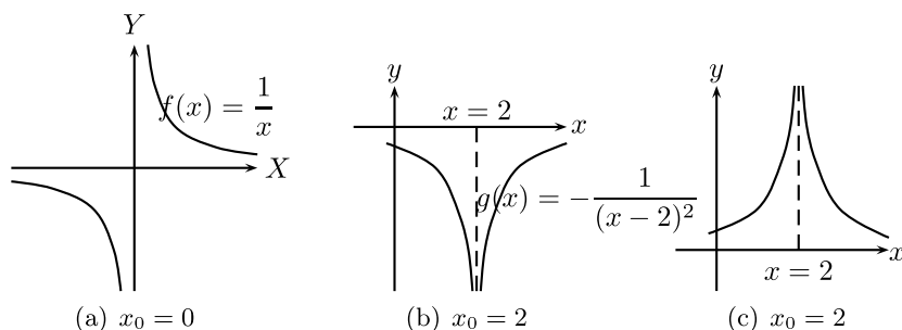
Figura 2.16: Comportamiento de algunas funciones cerca de puntos singulares.
