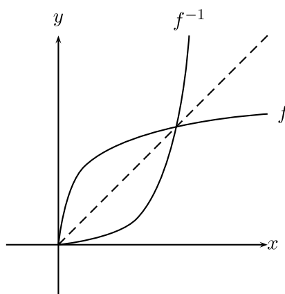
Figura 2.35: Continuidad de la inversa
