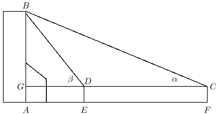
Figura 3.28: Torre de pie inaccesible
